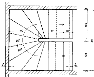
GRUNDRISS
