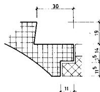
Schnitt B-B
