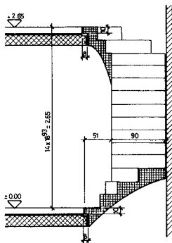
SCHNITT A-A
