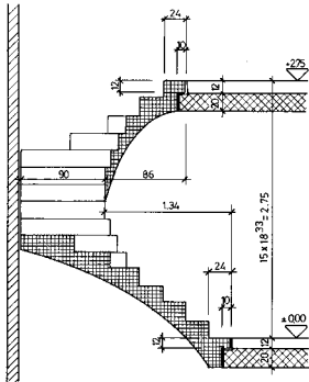
SCHNITT A-A
