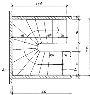
GRUNDRIS
